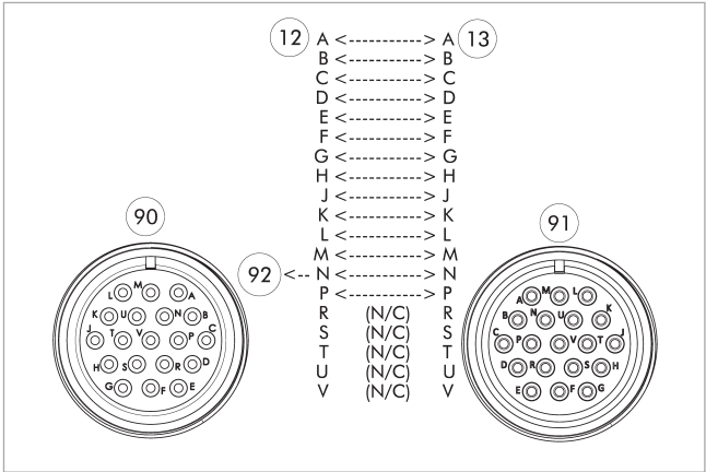
12 Côté maître 91 Prise femelle Amphenol MS, 19 contacts 13 Côté adaptateur 92 contact avancé 90 Prise mâle Amphenol MS, 19 contacts
