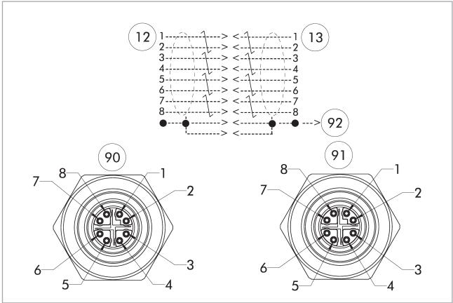
12 Côté maître 91 Prise femelle M12, codé X 13 Côté adaptateur 92 contact avancé 90 Prise femelle M12, codé X
